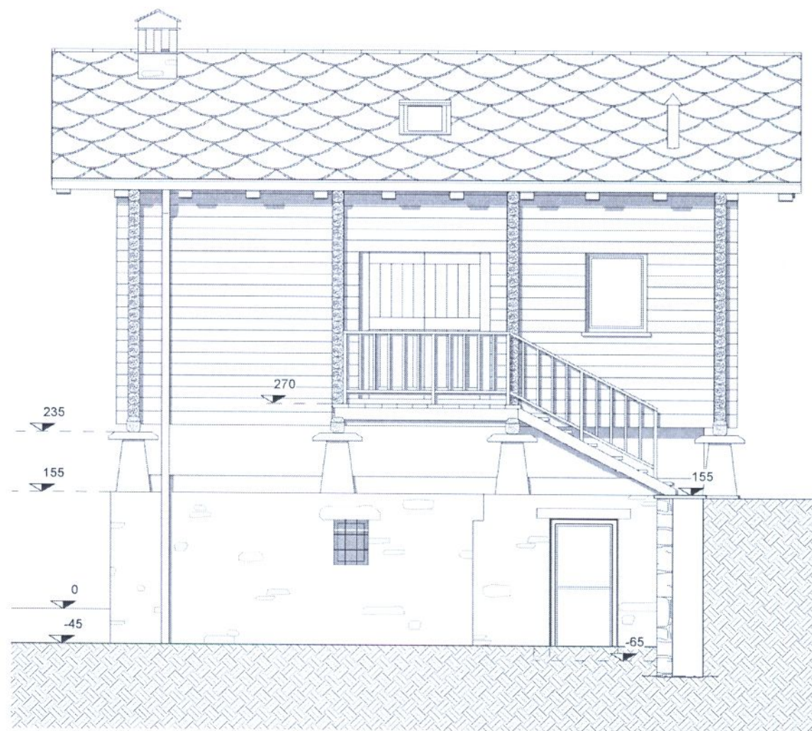
PROSPETTO SUD
