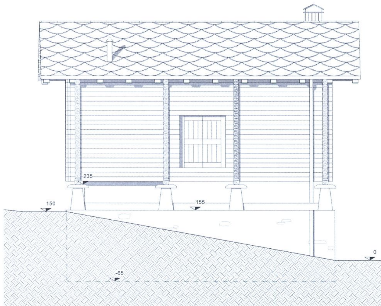
PROSPETTO NORD
