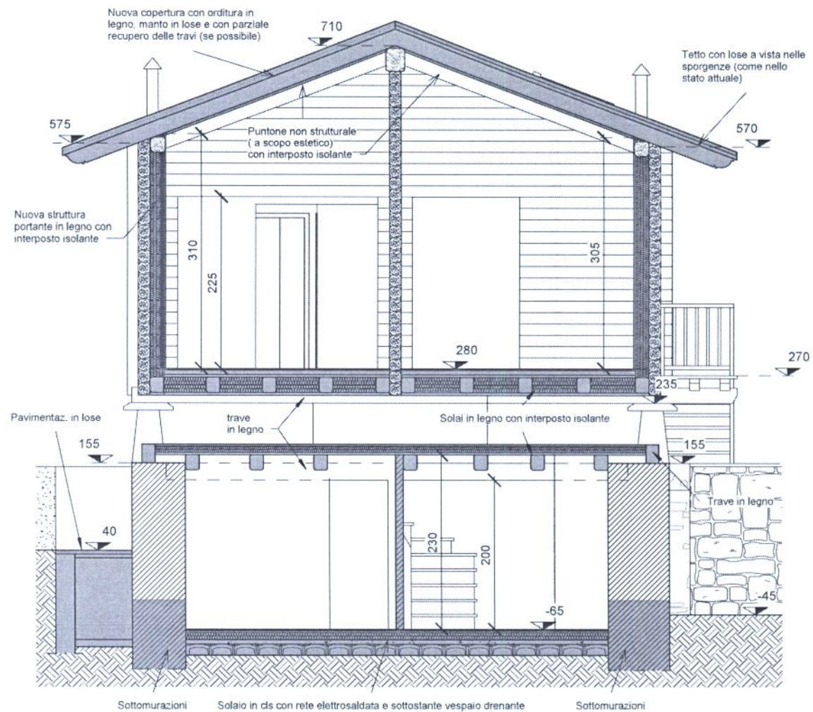
SEZIONE A-A'
