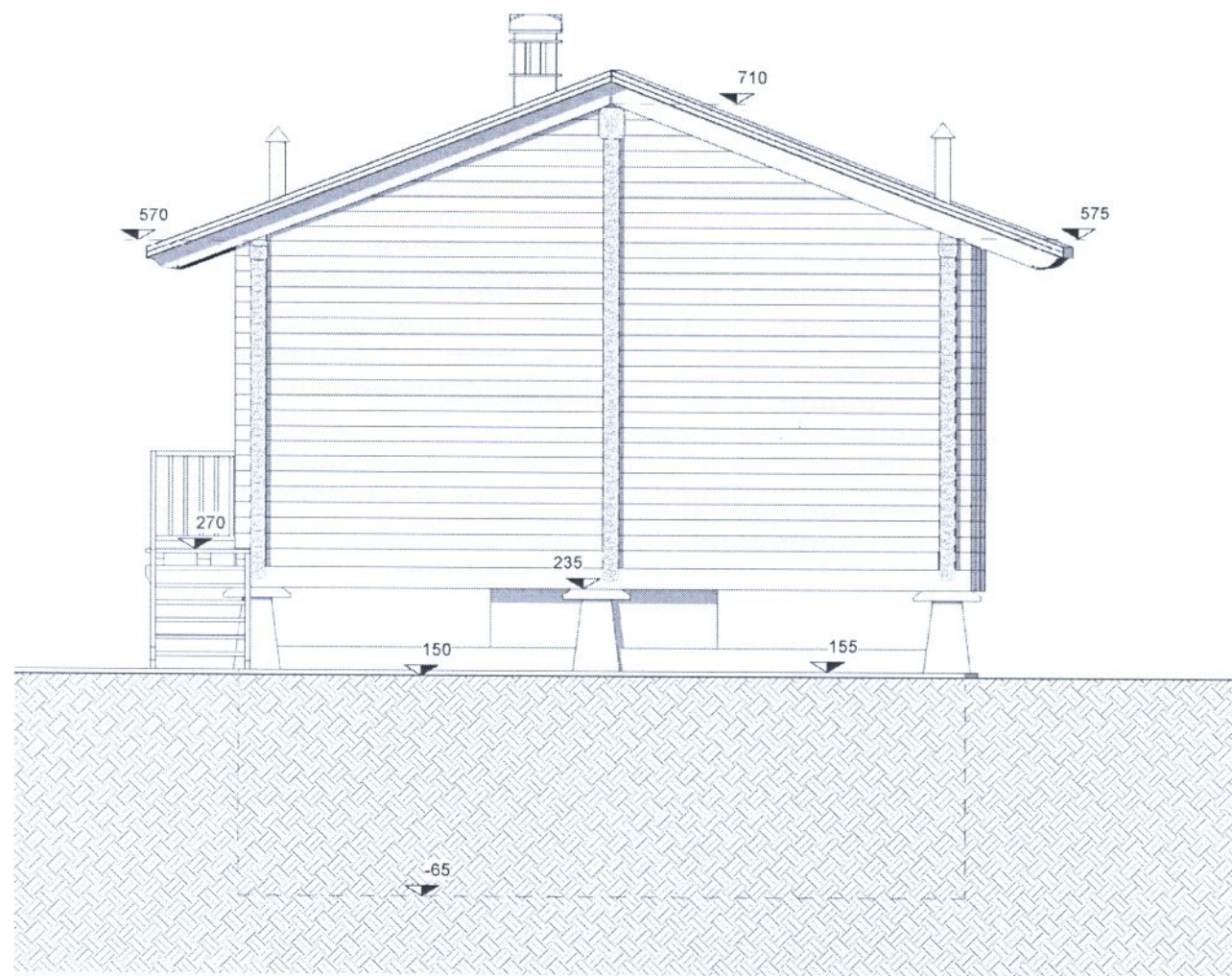
PROSPETTO EST
