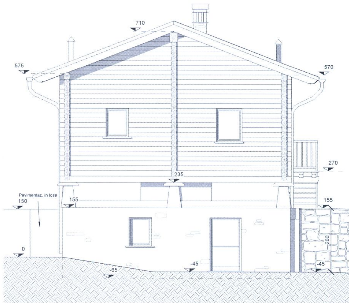
PROSPETTO OVEST
